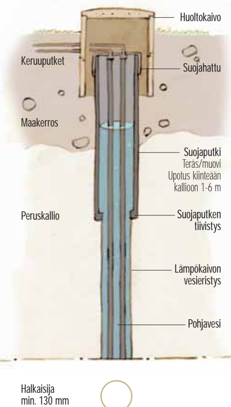
Porakaivon maksimisyvyys 200-250 m
